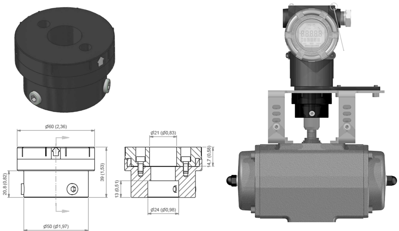
Figura 2.11 – Dimensional e montagem do ímã rotativo.
