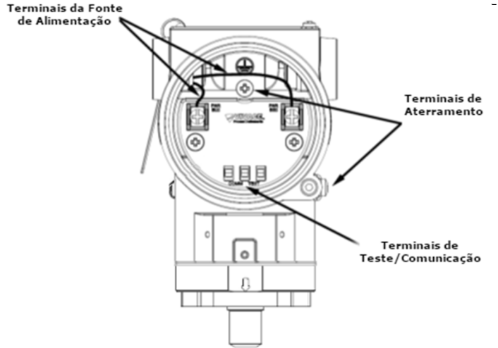
Figura 2.9 – Conexões e descrição dos terminais do VTP10-H.
