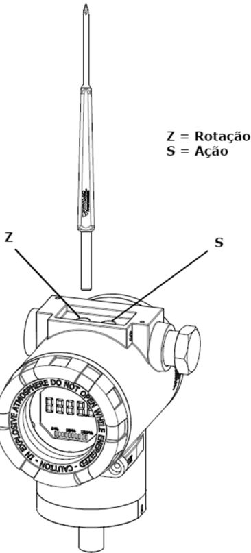
Figura 3.1 – Z e S do ajuste local e chave magnética.
